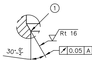
Einzelheit Y
