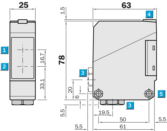
Габаритный чертеж (Размеры, мм)
