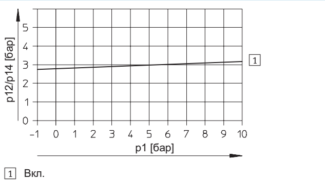
Минимальное пилотное давление p12/p14 как функция рабочего давления p1 (внешнее питание пилота)
