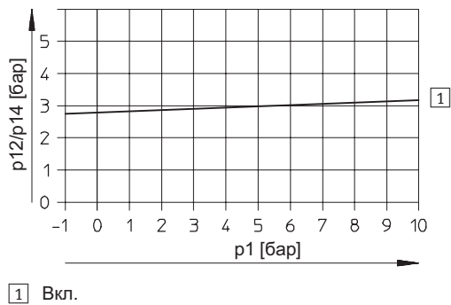
Минимальное пилотное давление p_{12/p14} как функция рабочего давления p_1 (внешнее питание пилота) MVH-5/3...-1/8-S-B MVH-5/3...-1/4-S-B
