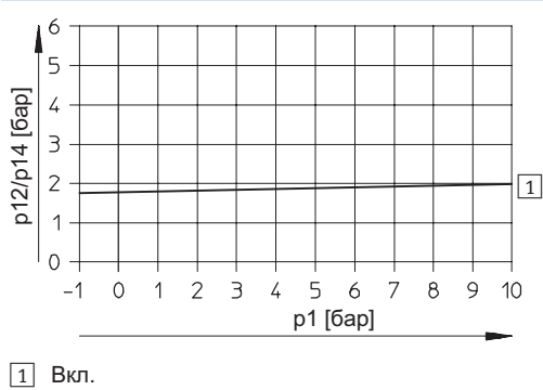
Минимальное пилотное давление p_{12/p14} как функция рабочего давления p_1 (внешнее питание пилота) JMFH-5-1/8-S-B JMFH-5-1/4-S-B
